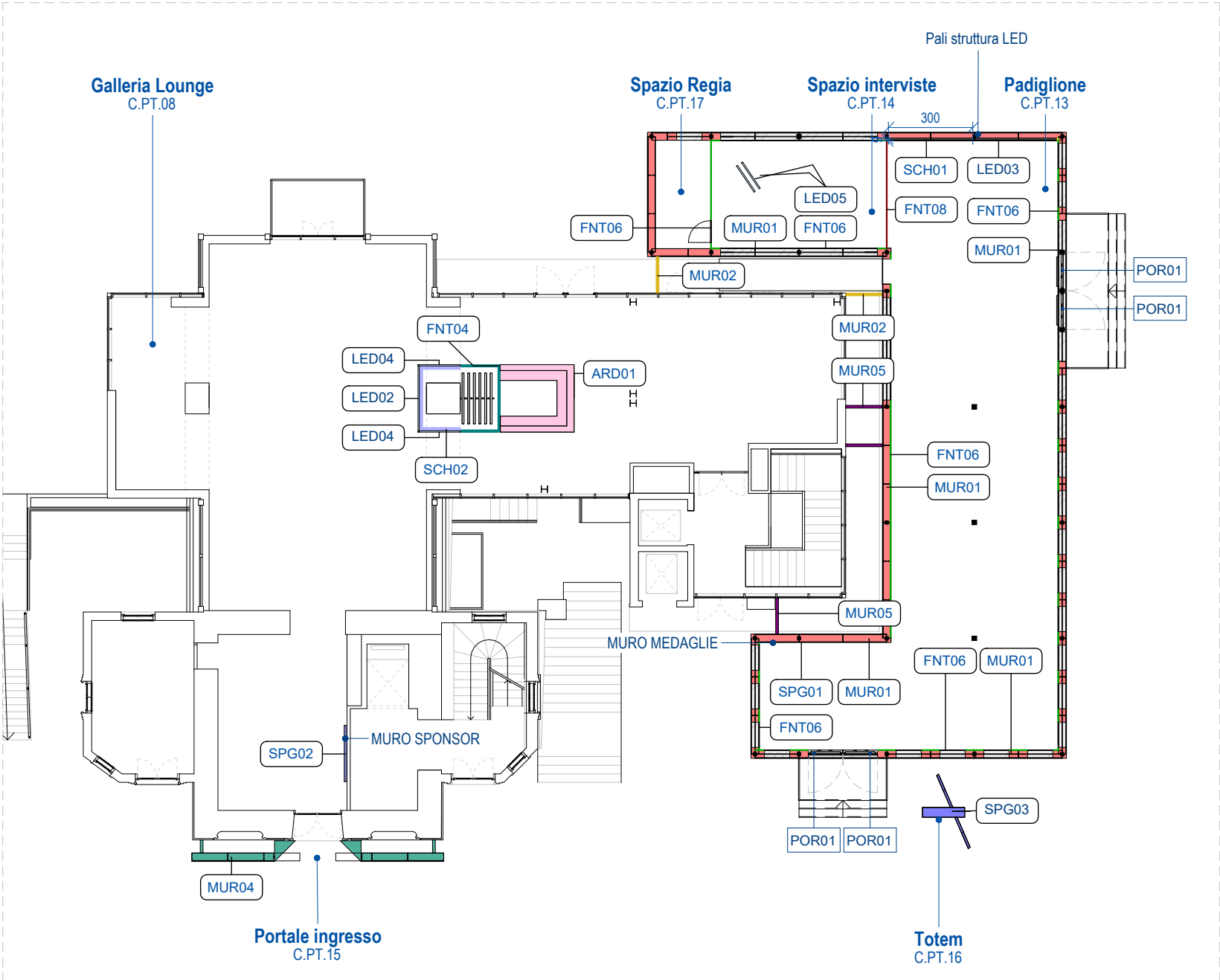
PIANTA PT - ABACO FINITURE VERTICALI 1 : 200
